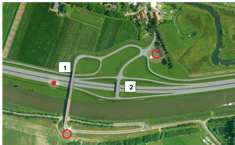
Afbeelding: Overzicht ontwerp ongelijkvloerse kruising Middelrode: 1 = verlenging Milrooijsbrug, 2 = nieuw viaduct N279
